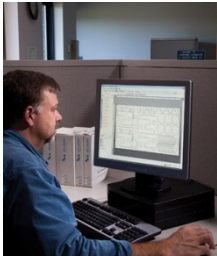
ProNest 2010
